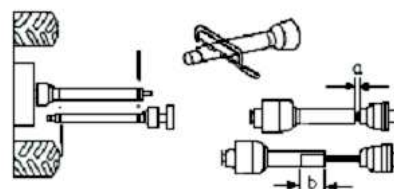
Рисунок 4: Укорачивание приводного вала механизма отбора мощности
