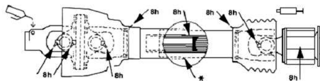
Рис. 9 Смазка приводного вала
